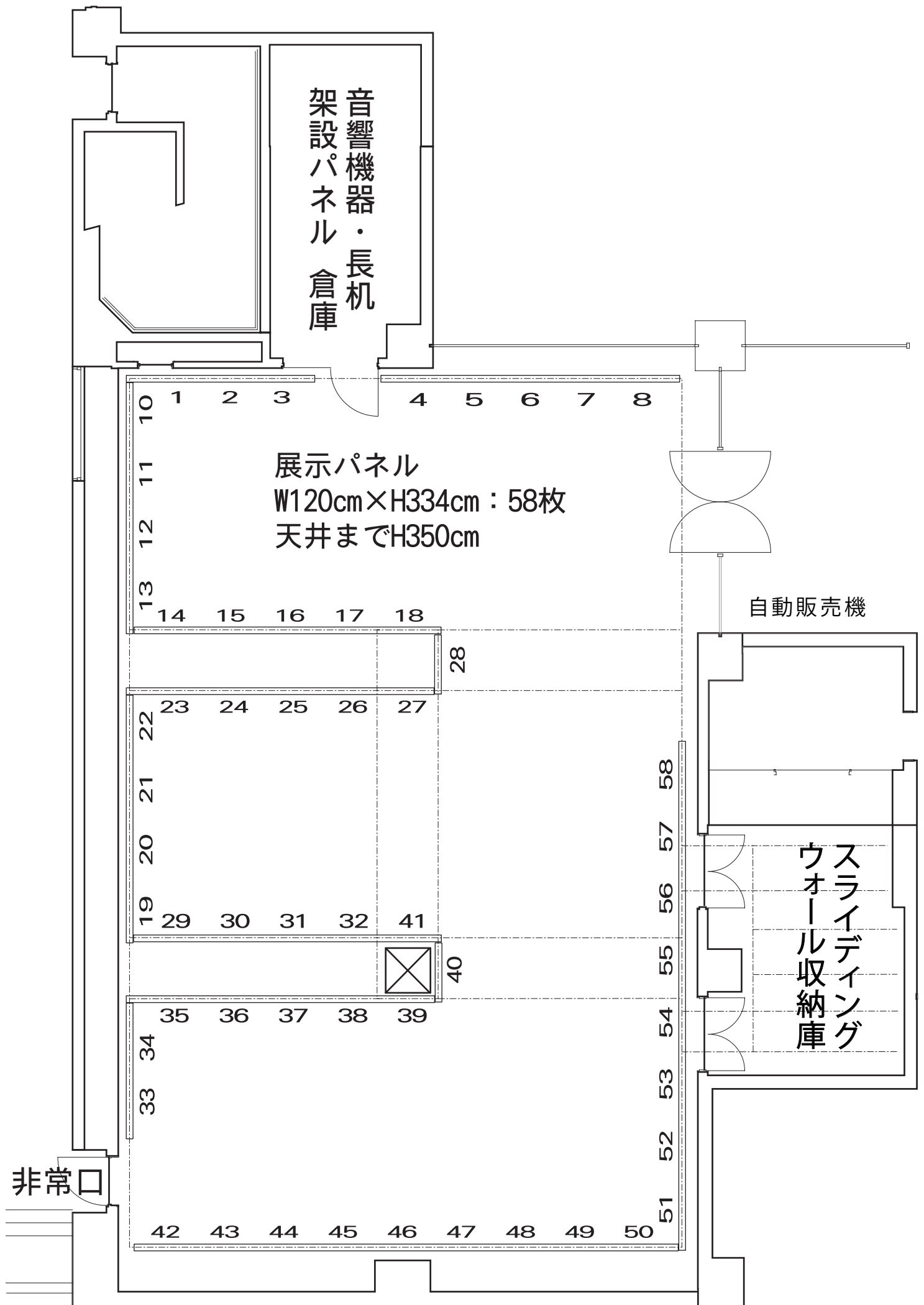
安芸区民文化センター 1階 ギャラリー パネル設営図
