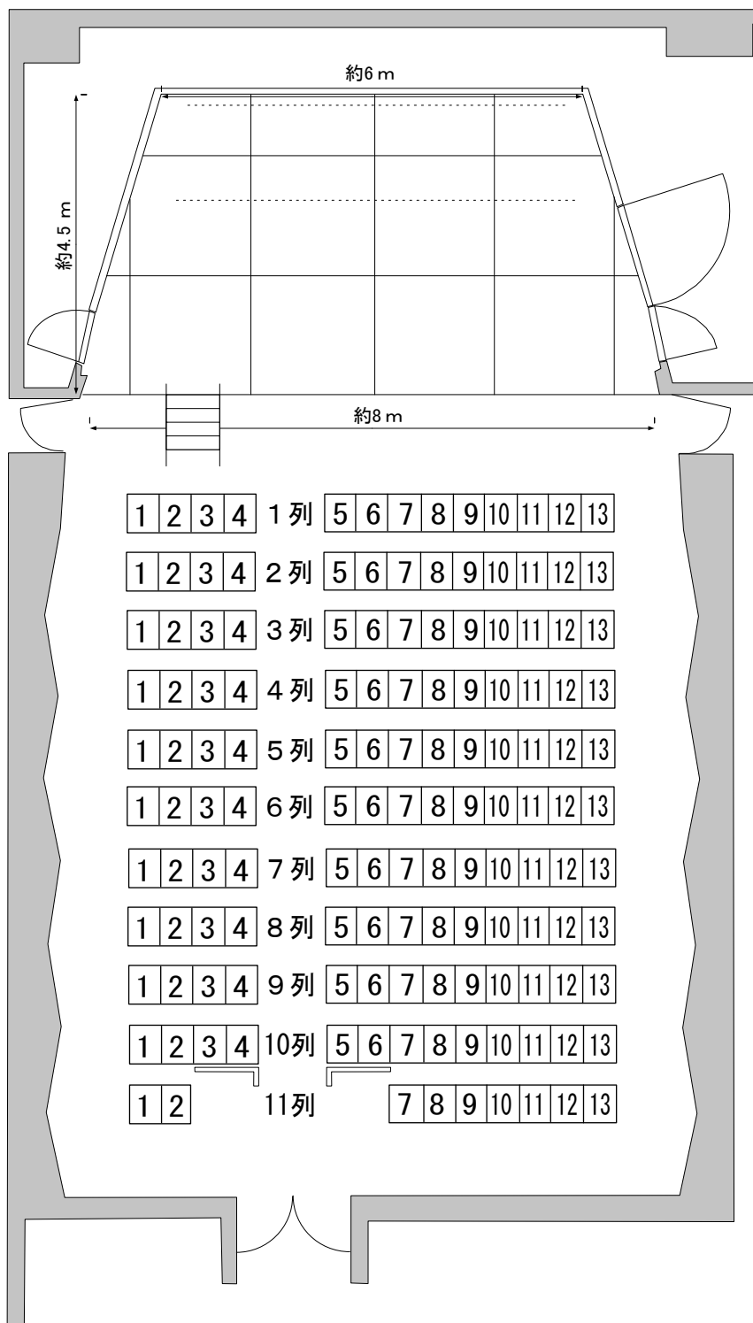
舞台・客席平面図 (S 1 : 100)
