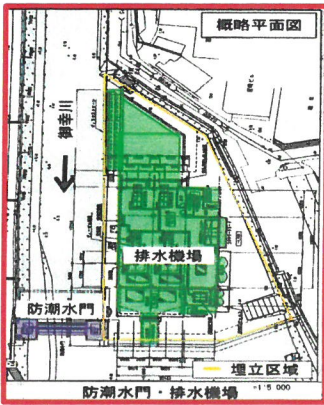
防潮水門・排水機場 設置拡大図
