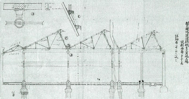
製缶場護謨機械室及其他工場縦断面図 青図を反転 当館蔵
