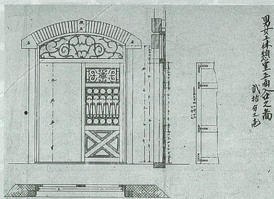
男女工休憩室正面入口之図 青図を反転 当館蔵
