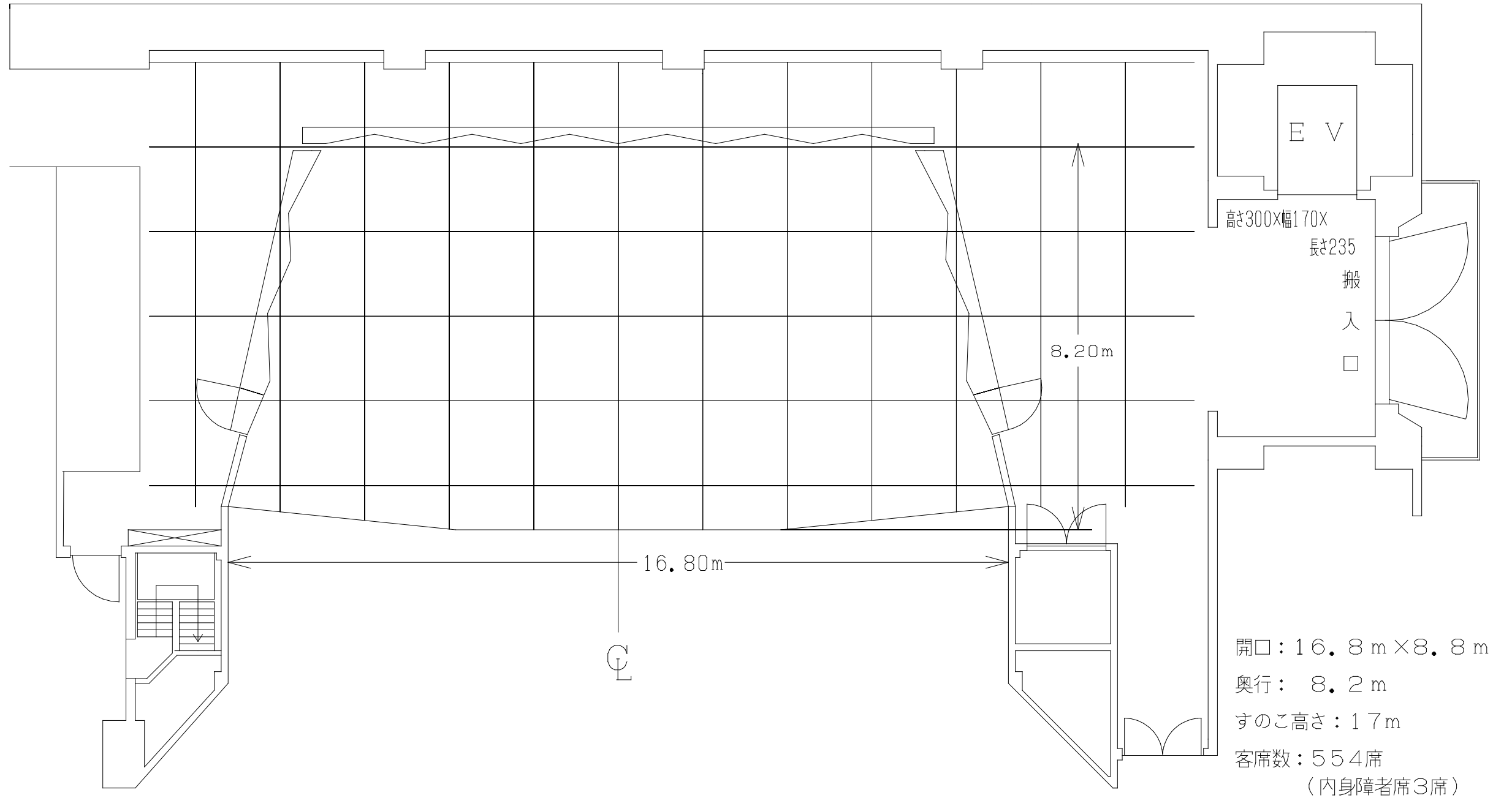
南区民文化センター舞台平面図 (S=1:100)
